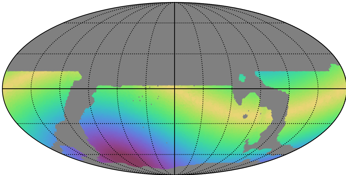
weather_cloudso36v3.4_10yrs WFD y band: Max solarElong
