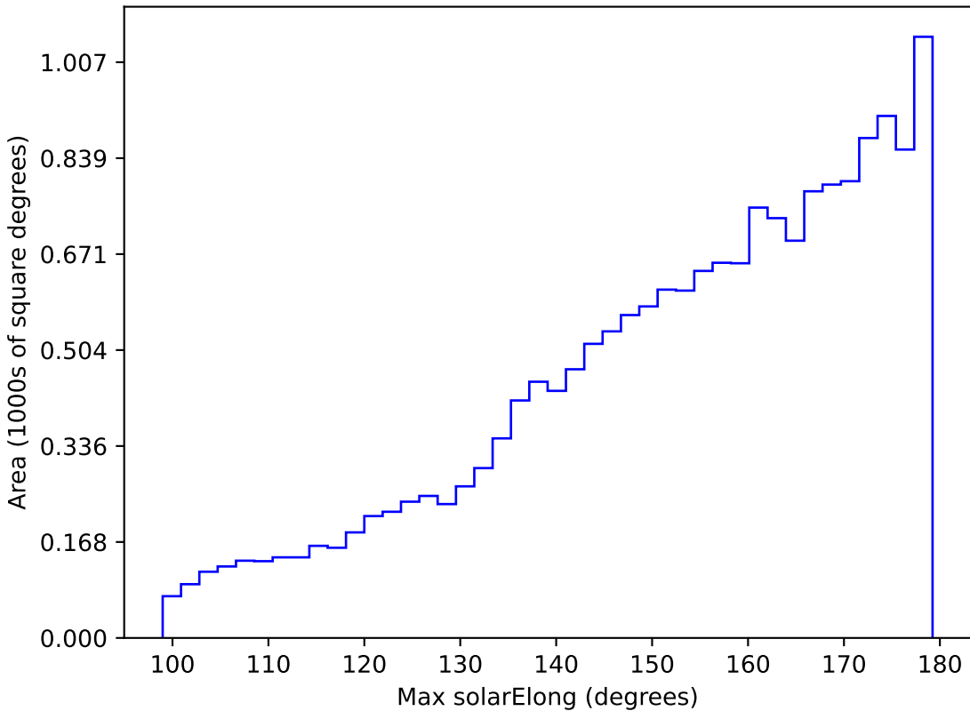
weather_cloudso36v3.4_10yrs WFD y band: Max solarElong
