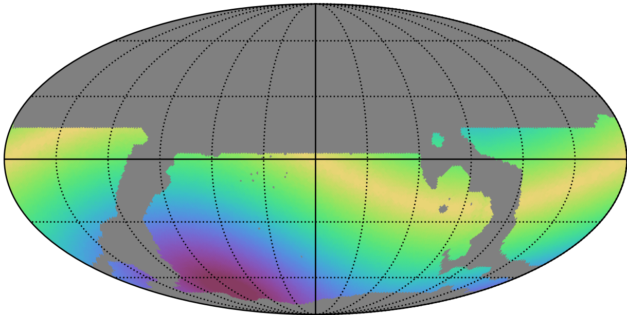
weather_cloudso36v3.4_10yrs WFD i band: Max solarElong
