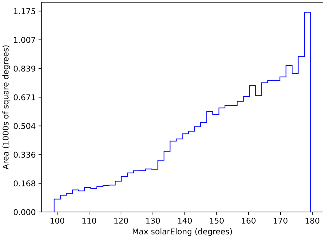
weather_cloudso36v3.4_10yrs WFD i band: Max solarElong
