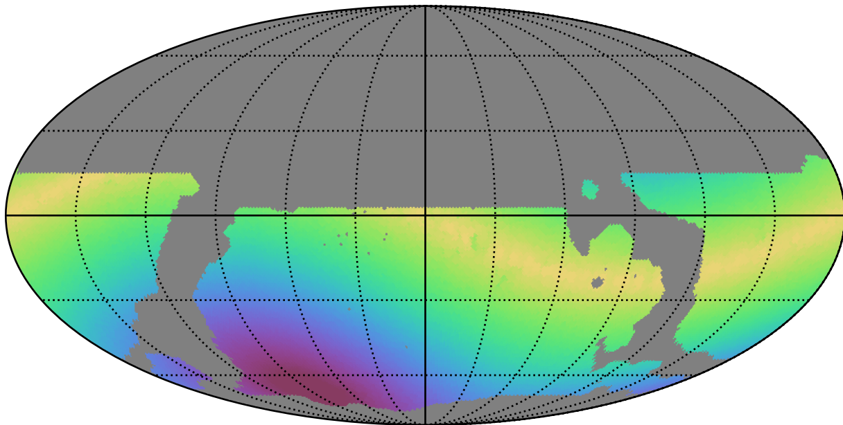
weather_cloudso36v3.4_10yrs WFD g band: Max solarElong
