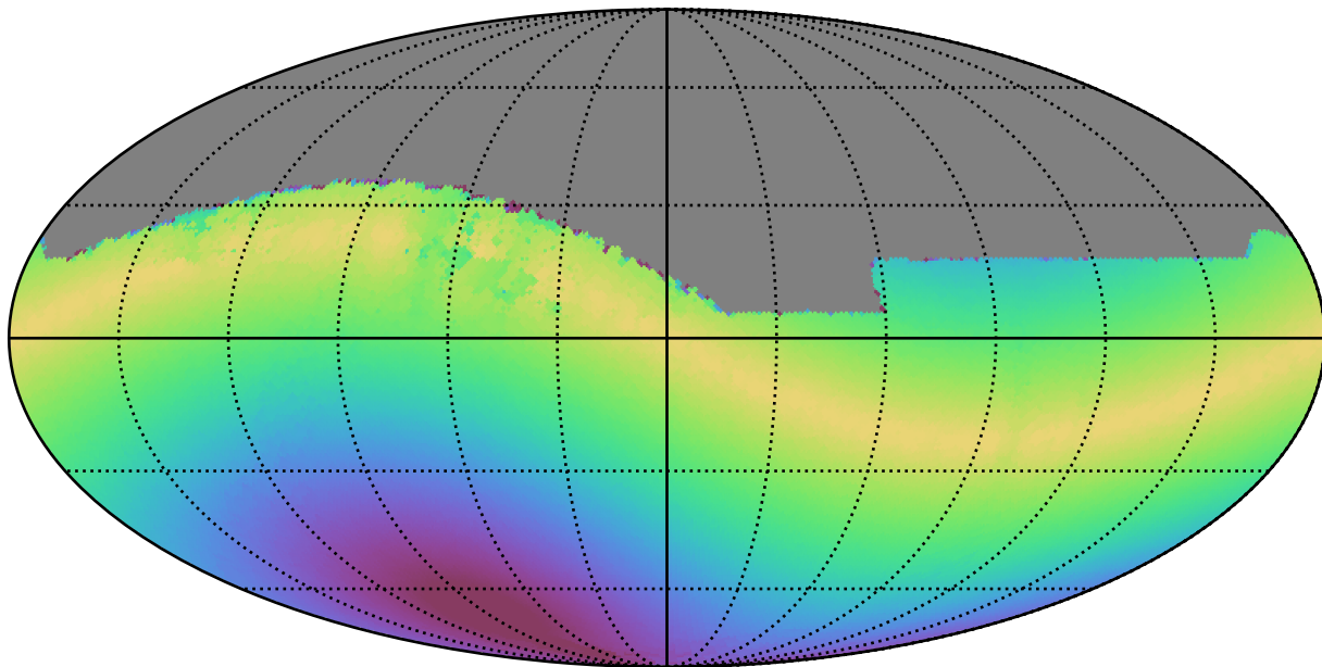
weather_cloudso36v3.4_10yrs All sky z band: Max solarElong
