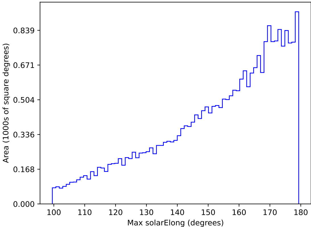
weather_cloudso36v3.4_10yrs All sky z band: Max solarElong
