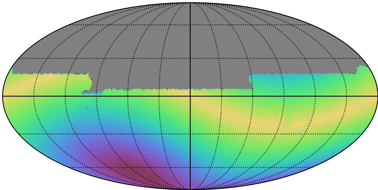
weather_cloudso36v3.4_10yrs All sky y band: Max solarElong
