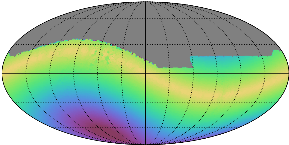
weather_cloudso36v3.4_10yrs All sky i band: Max solarElong
