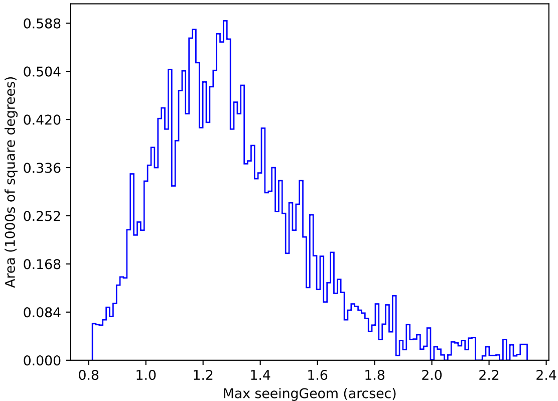
weather_cloudso36v3.4_10yrs Yr 1 y band: Max seeingGeom
