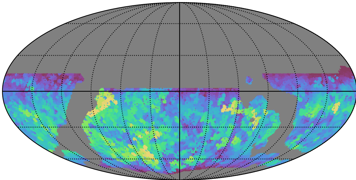
weather_cloudso36v3.4_10yrs WFD z band: Max saturation_mag
