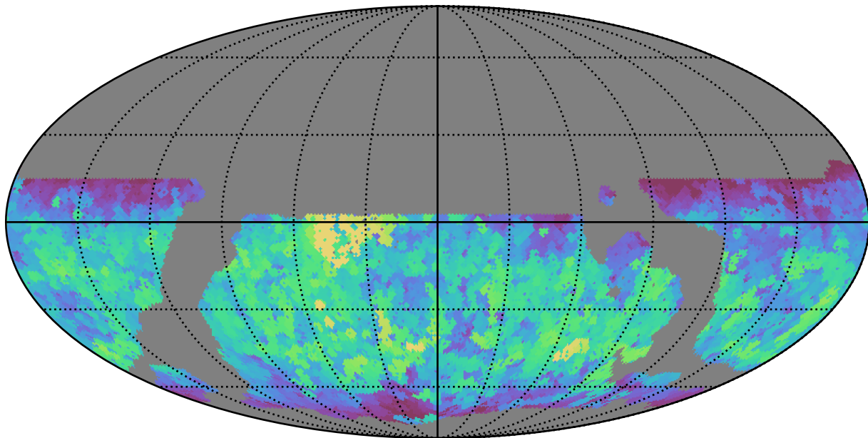
weather_cloudso36v3.4_10yrs WFD y band: Max saturation_mag
