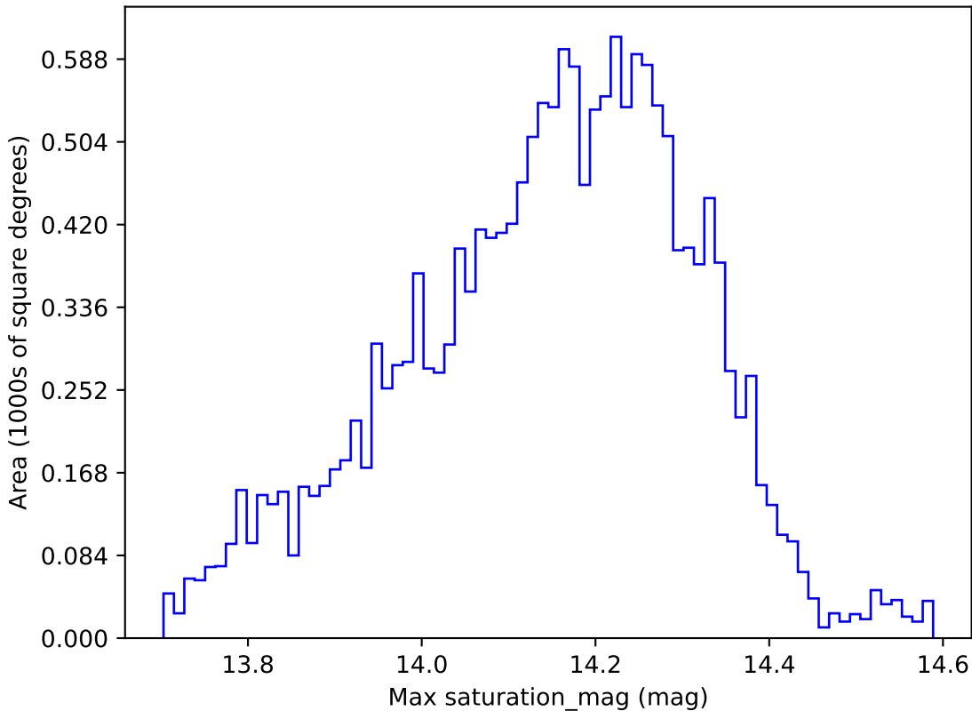
weather_cloudso36v3.4_10yrs WFD y band: Max saturation_mag
