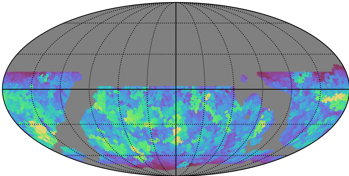
weather_cloudso36v3.4_10yrs WFD r band: Max saturation_mag
