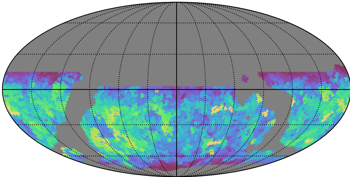
weather_cloudso36v3.4_10yrs WFD i band: Max saturation_mag
