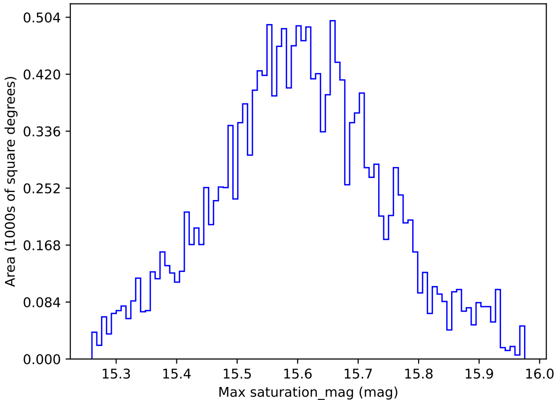
weather_cloudso36v3.4_10yrs WFD i band: Max saturation_mag
