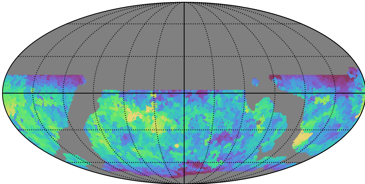
weather_cloudso36v3.4_10yrs WFD g band: Max saturation_mag
