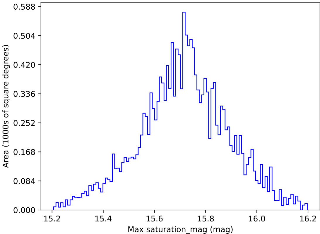
weather_cloudso36v3.4_10yrs WFD g band: Max saturation_mag
