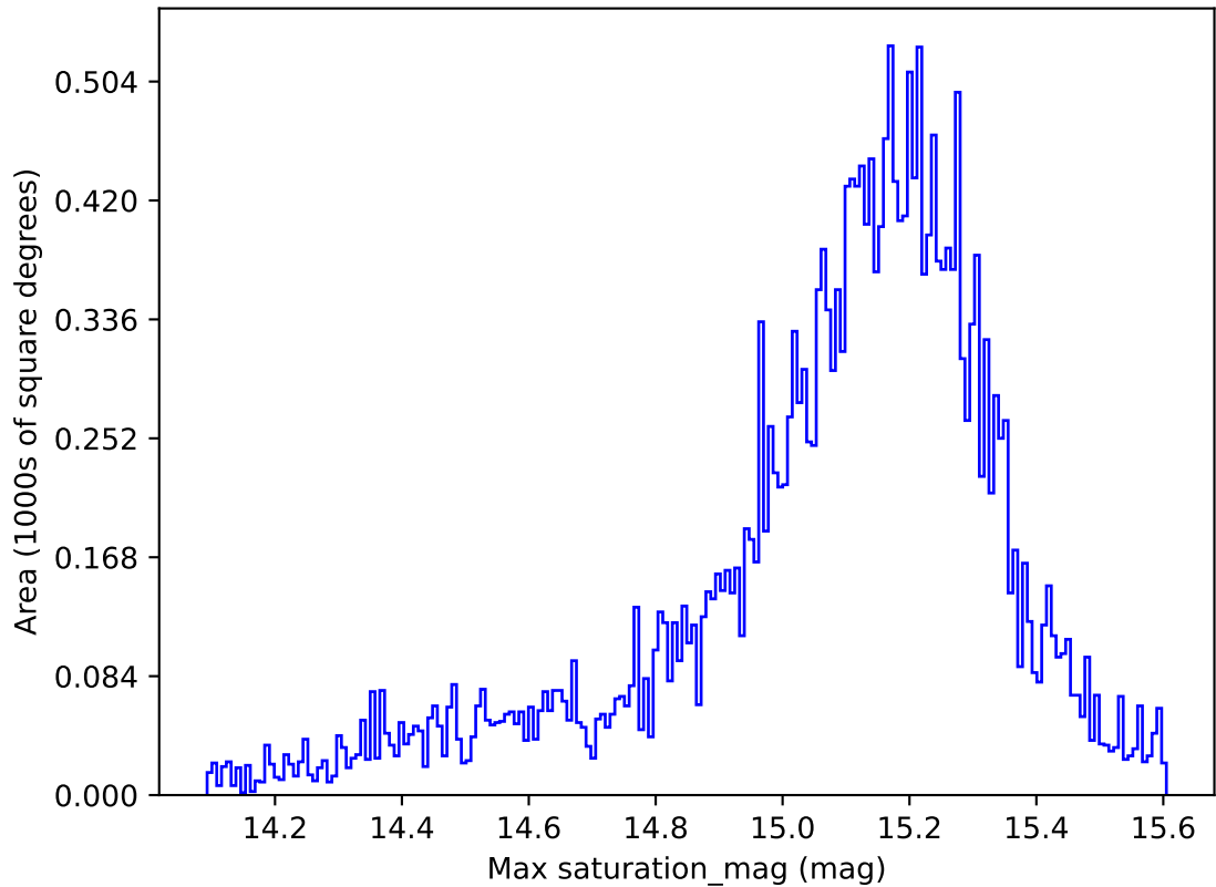
weather_cloudso36v3.4_10yrs All sky z band: Max saturation_mag
