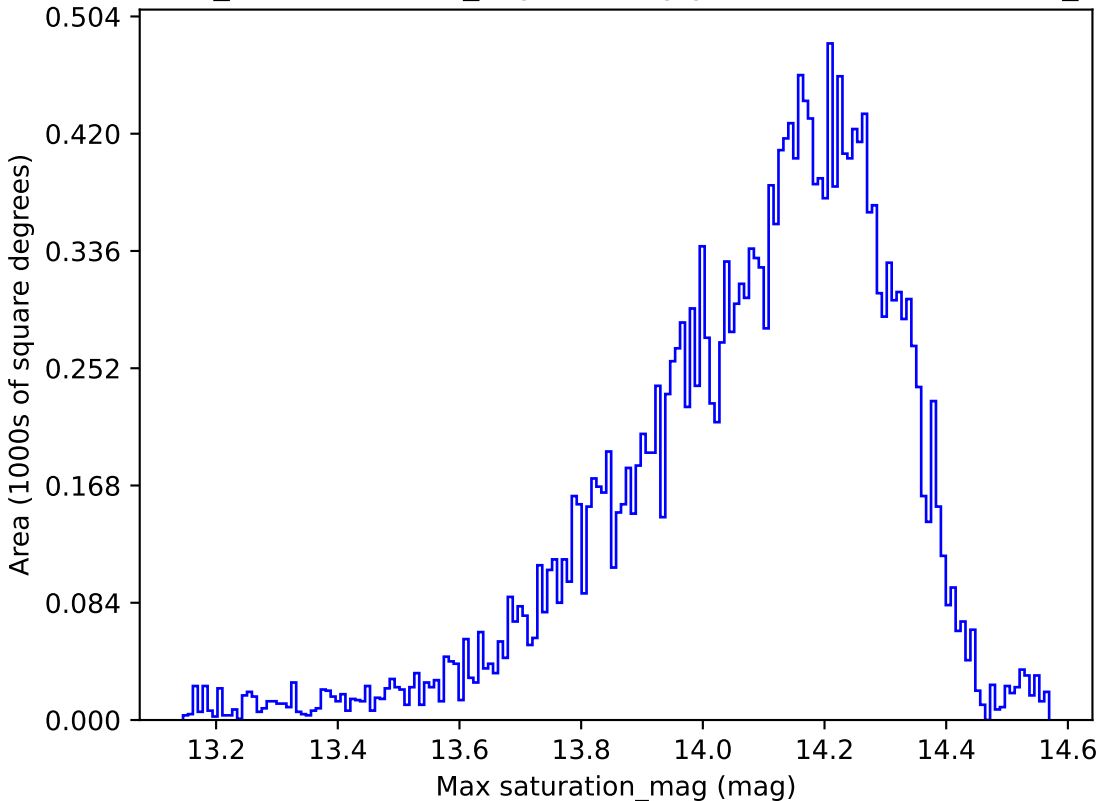
weather_cloudso36v3.4_10yrs All sky y band: Max saturation_mag
