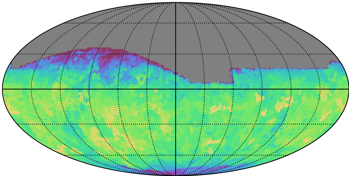
weather_cloudso36v3.4_10yrs All sky i band: Max saturation_mag
