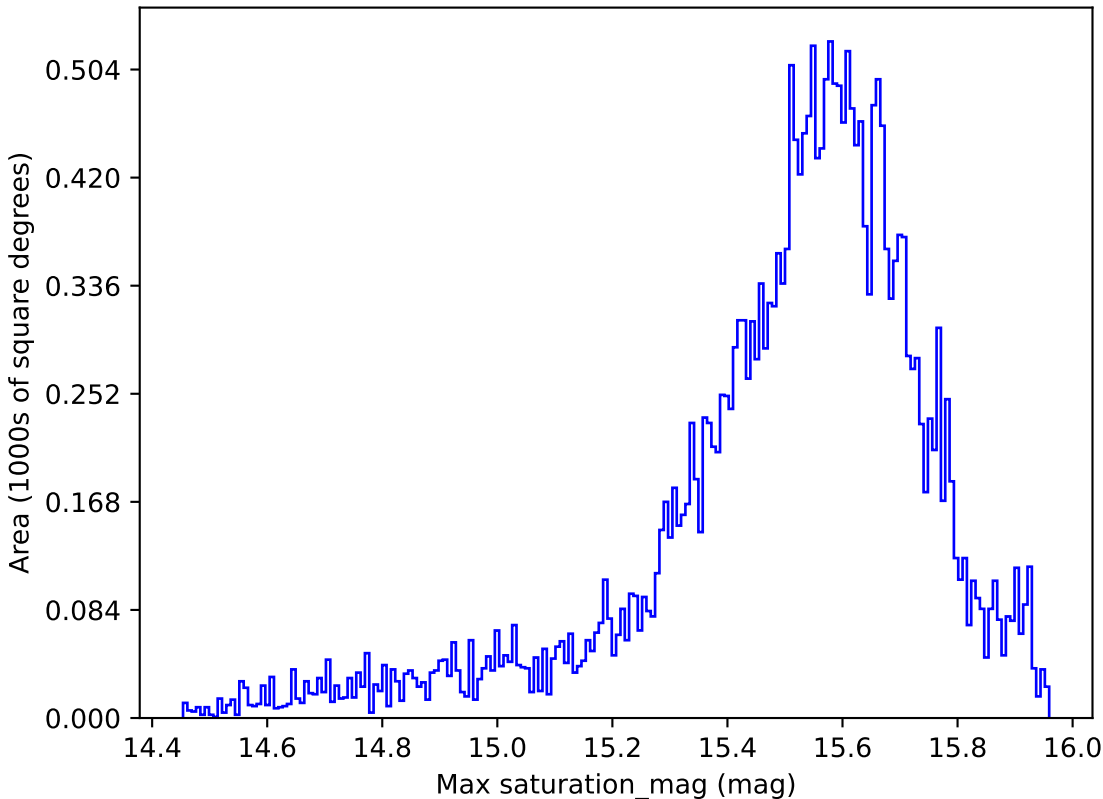
weather_cloudso36v3.4_10yrs All sky i band: Max saturation_mag
