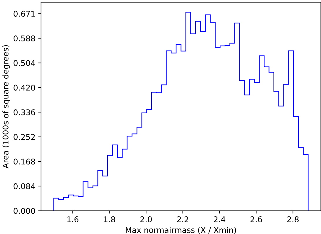
weather_cloudso36v3.4_10yrs WFD z band: Max normairmass
