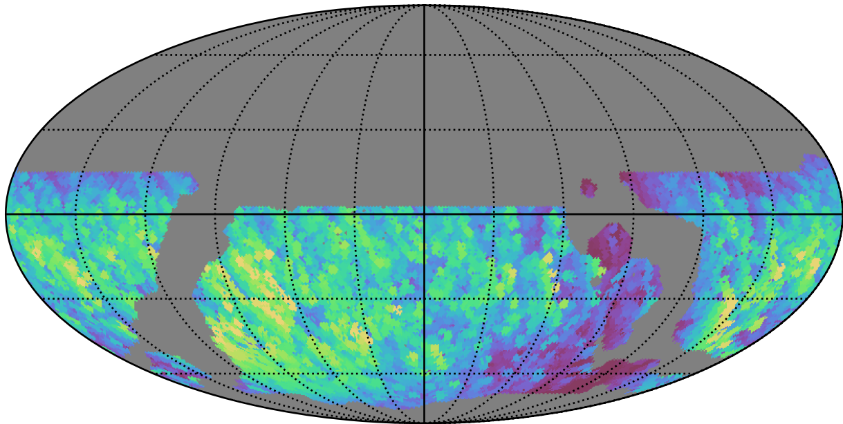
weather_cloudso36v3.4_10yrs WFD y band: Max normairmass
