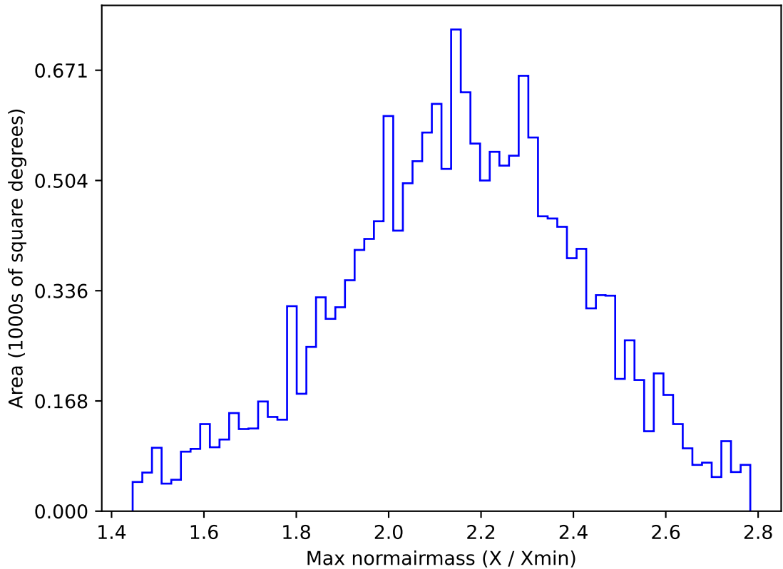
weather_cloudso36v3.4_10yrs WFD y band: Max normairmass
