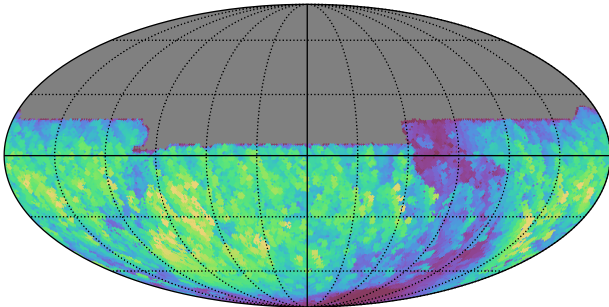
weather_cloudso36v3.4_10yrs All sky y band: Max normairmass
