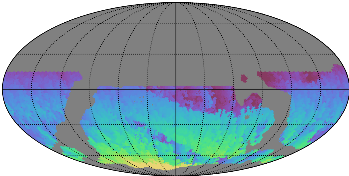
weather_cloudso36v3.4_10yrs WFD z band: Max HA
