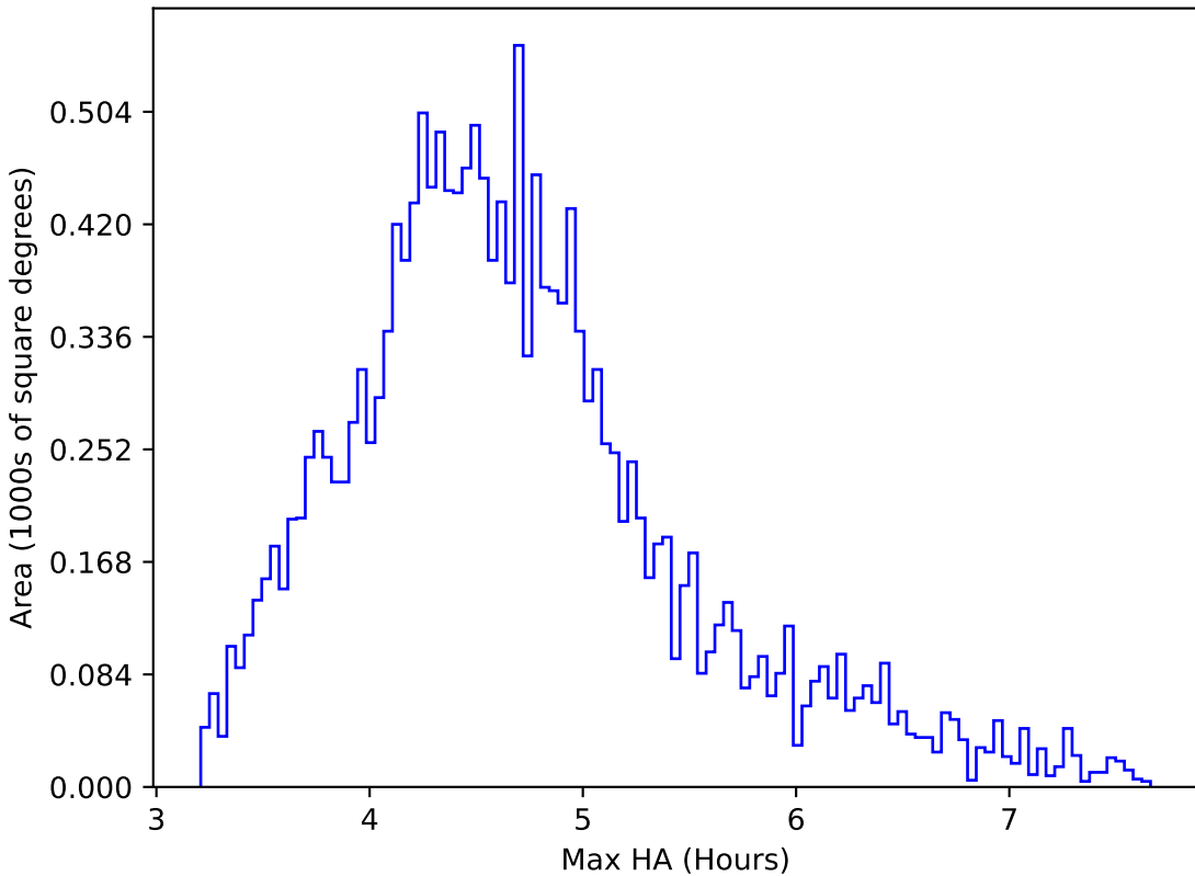
weather_cloudso36v3.4_10yrs WFD y band: Max HA
