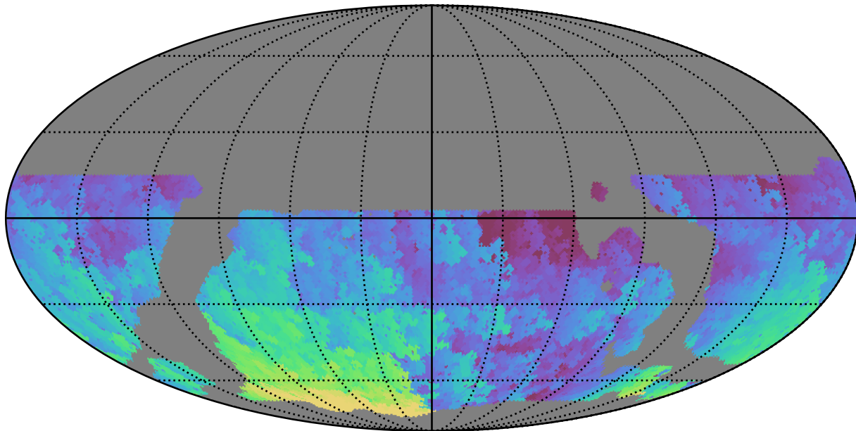
weather_cloudso36v3.4_10yrs WFD u band: Max HA
