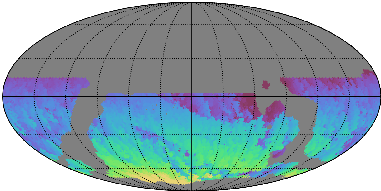
weather_cloudso36v3.4_10yrs WFD i band: Max HA
