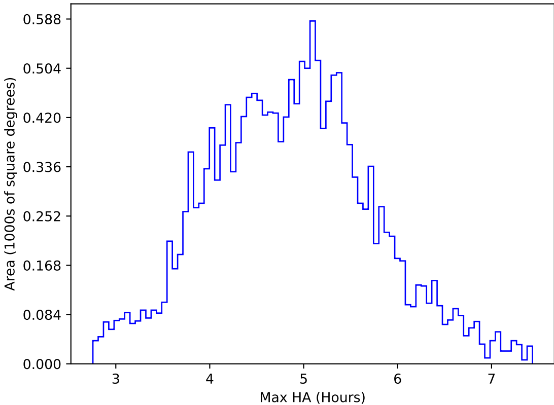
weather_cloudso36v3.4_10yrs WFD i band: Max HA
