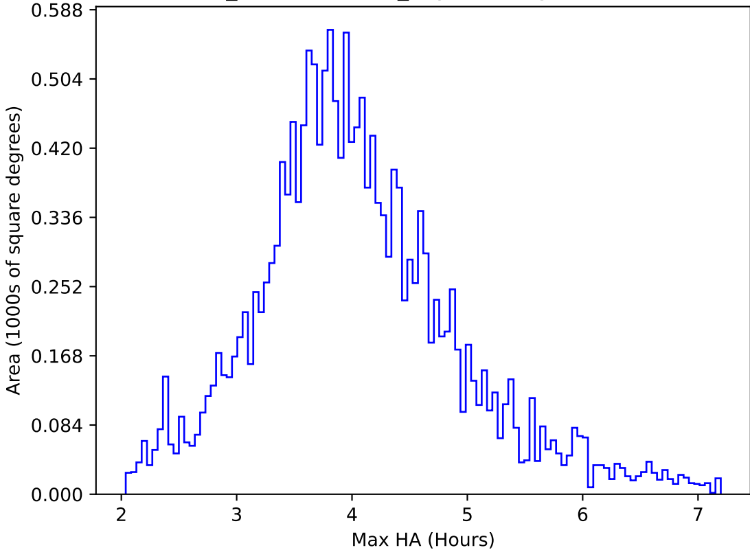
weather_cloudso36v3.4_10yrs WFD g band: Max HA
