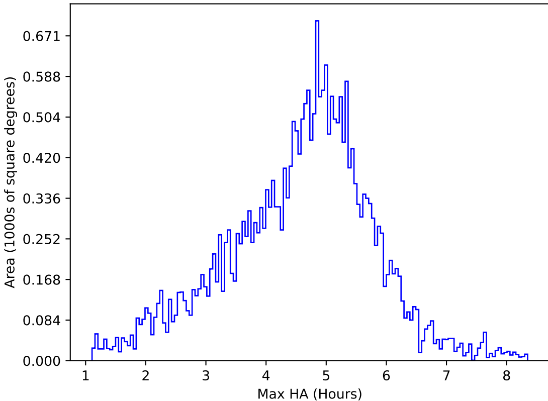
weather_cloudso36v3.4_10yrs All sky z band: Max HA
