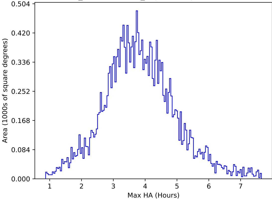
weather_cloudso36v3.4_10yrs All sky u band: Max HA
