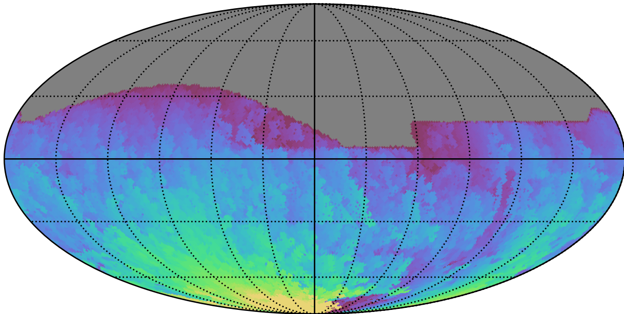
weather_cloudso36v3.4_10yrs All sky r band: Max HA
