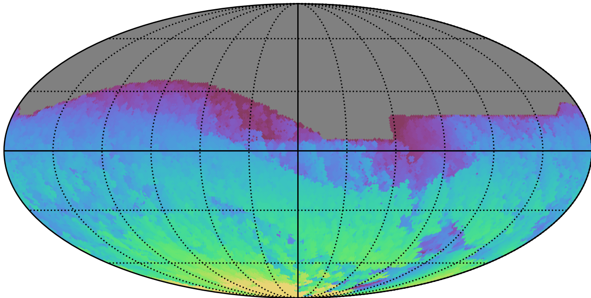
weather_cloudso36v3.4_10yrs All sky i band: Max HA
