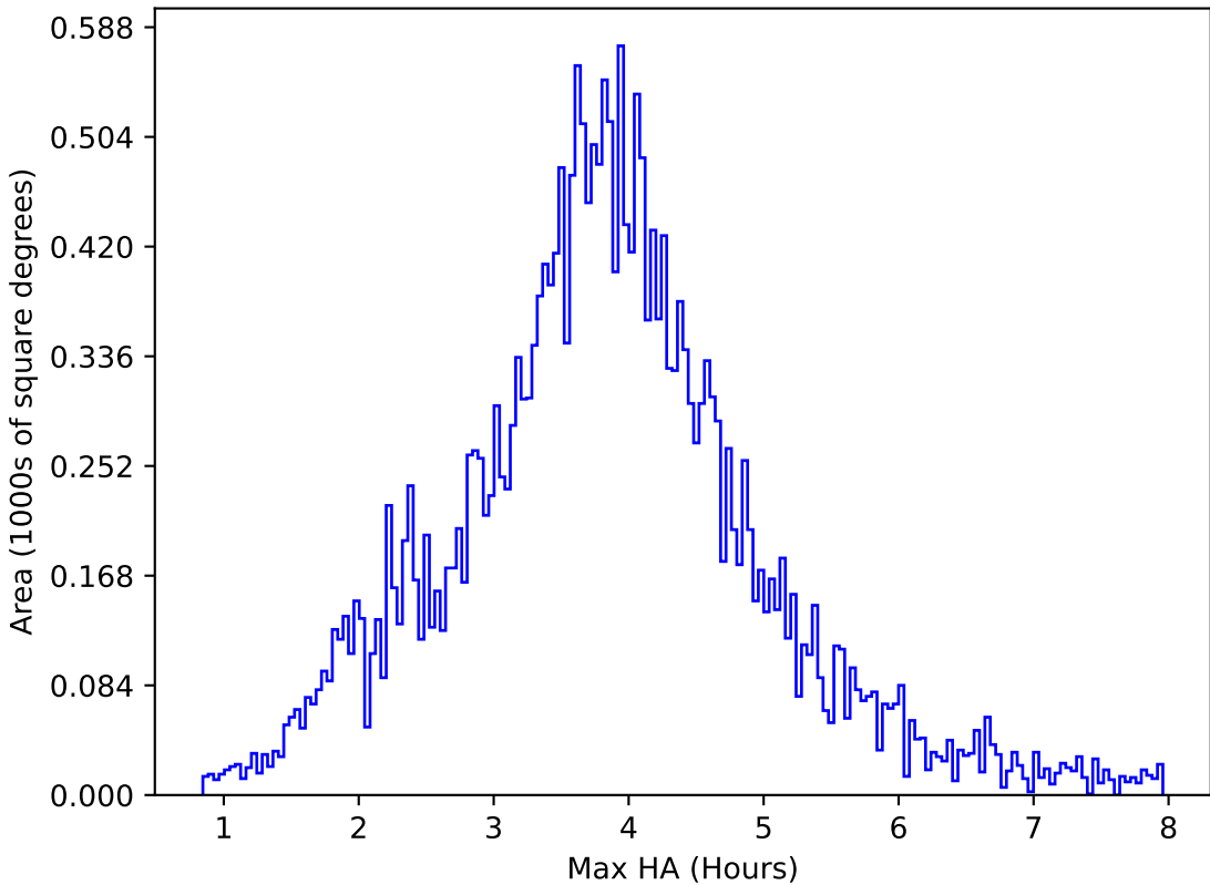
weather_cloudso36v3.4_10yrs All sky g band: Max HA
