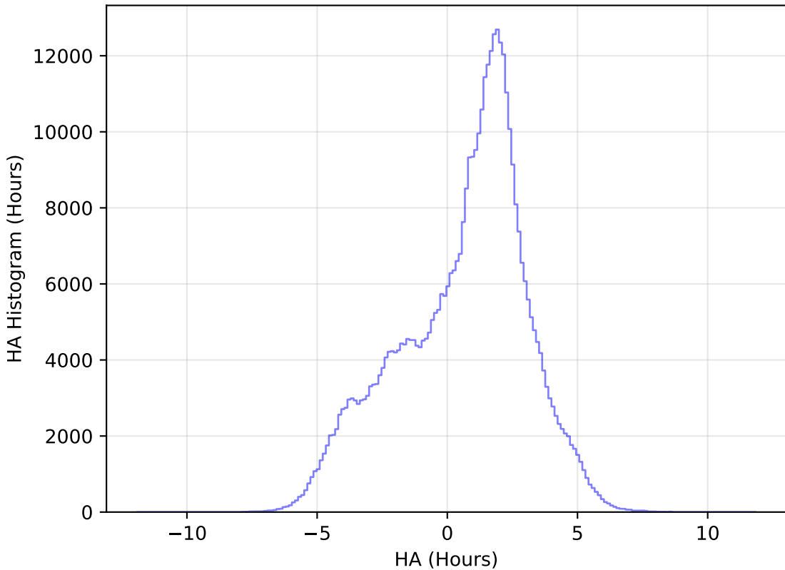
weather_cloudso36v3.4_10yrs WFD z band: HA Histogram
