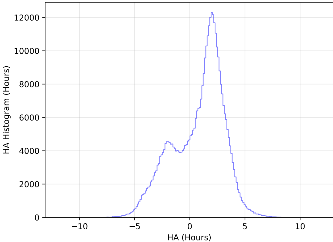
weather_cloudso36v3.4_10yrs WFD y band: HA Histogram
