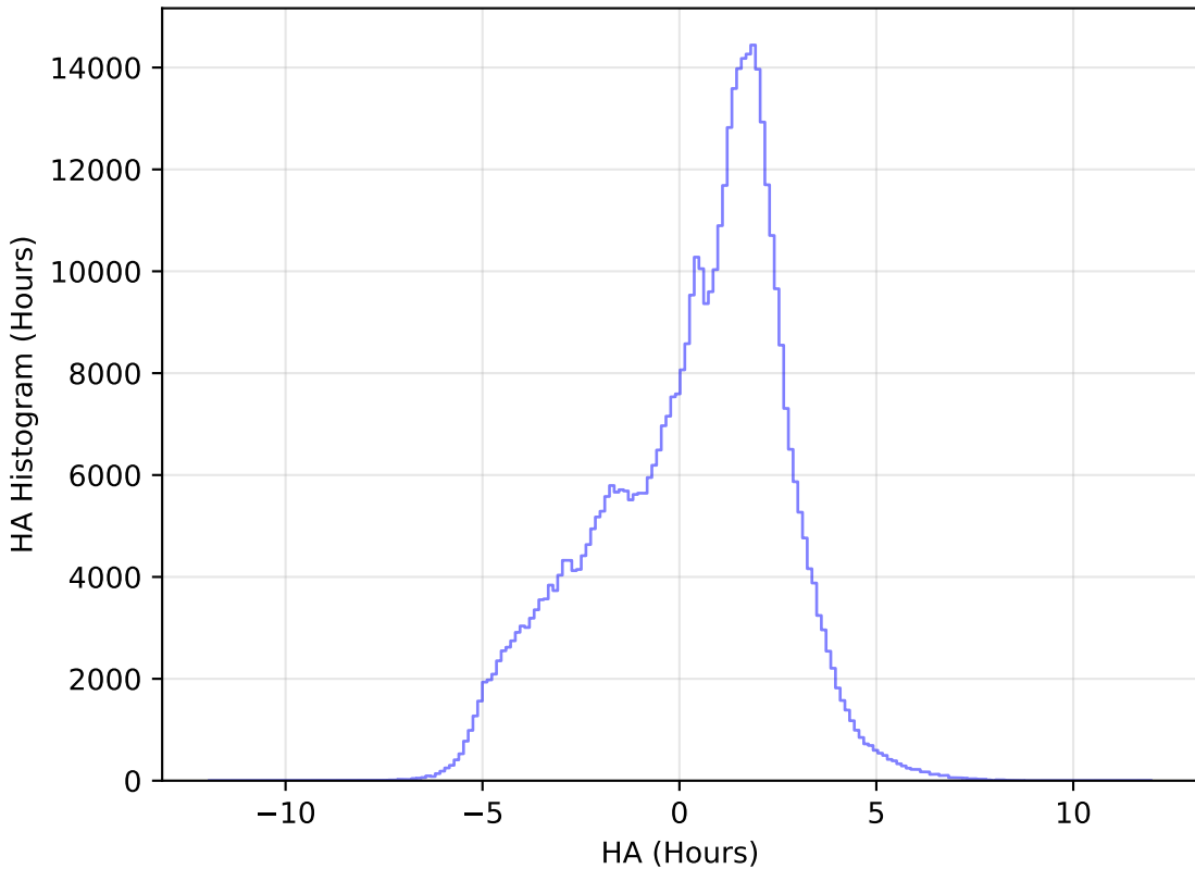
weather_cloudso36v3.4_10yrs WFD r band: HA Histogram
