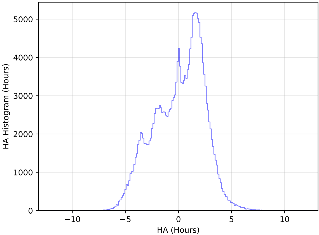
weather_cloudso36v3.4_10yrs WFD g band: HA Histogram
