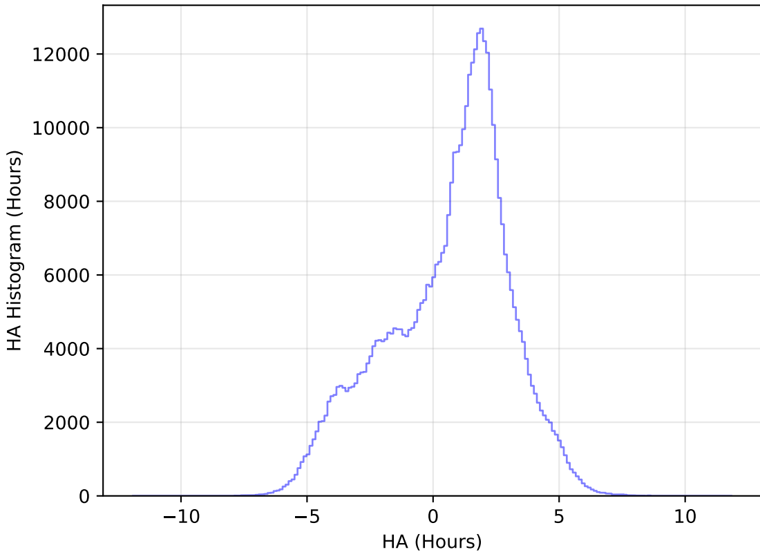
weather_cloudso36v3.4_10yrs All sky z band: HA Histogram
