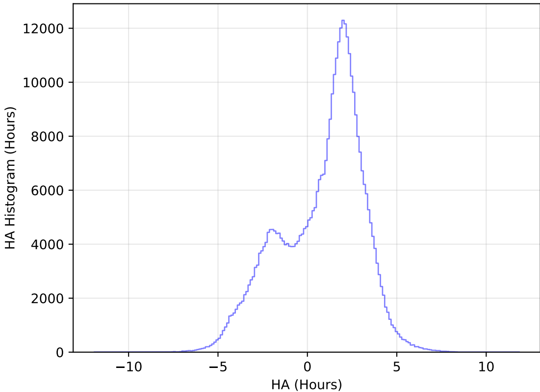
weather_cloudso36v3.4_10yrs All sky y band: HA Histogram
