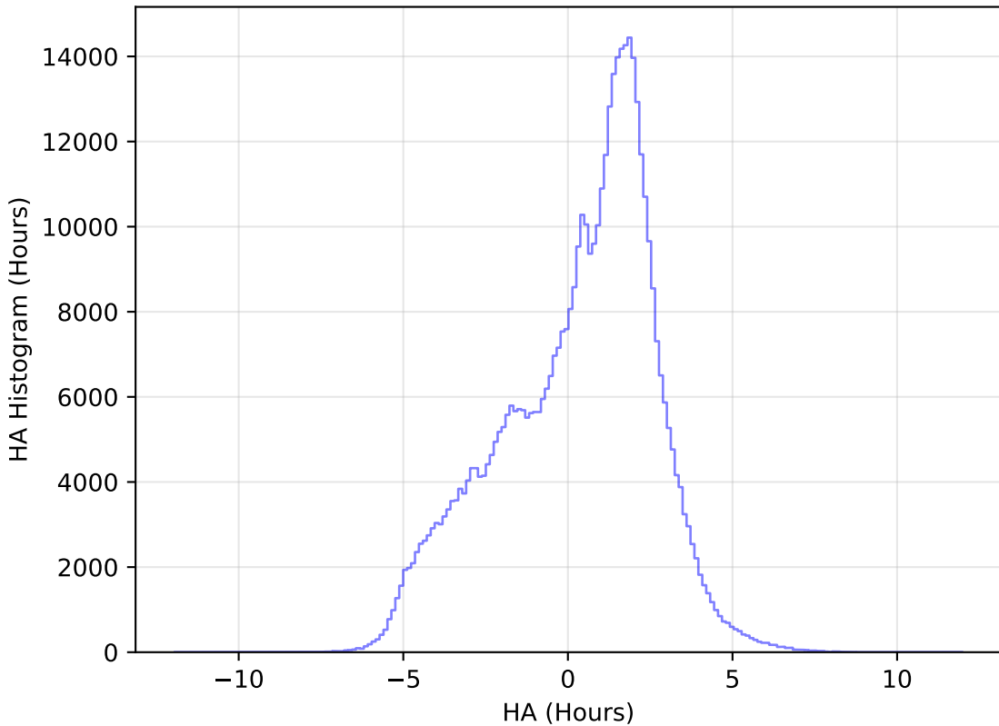
weather_cloudso36v3.4_10yrs All sky r band: HA Histogram
