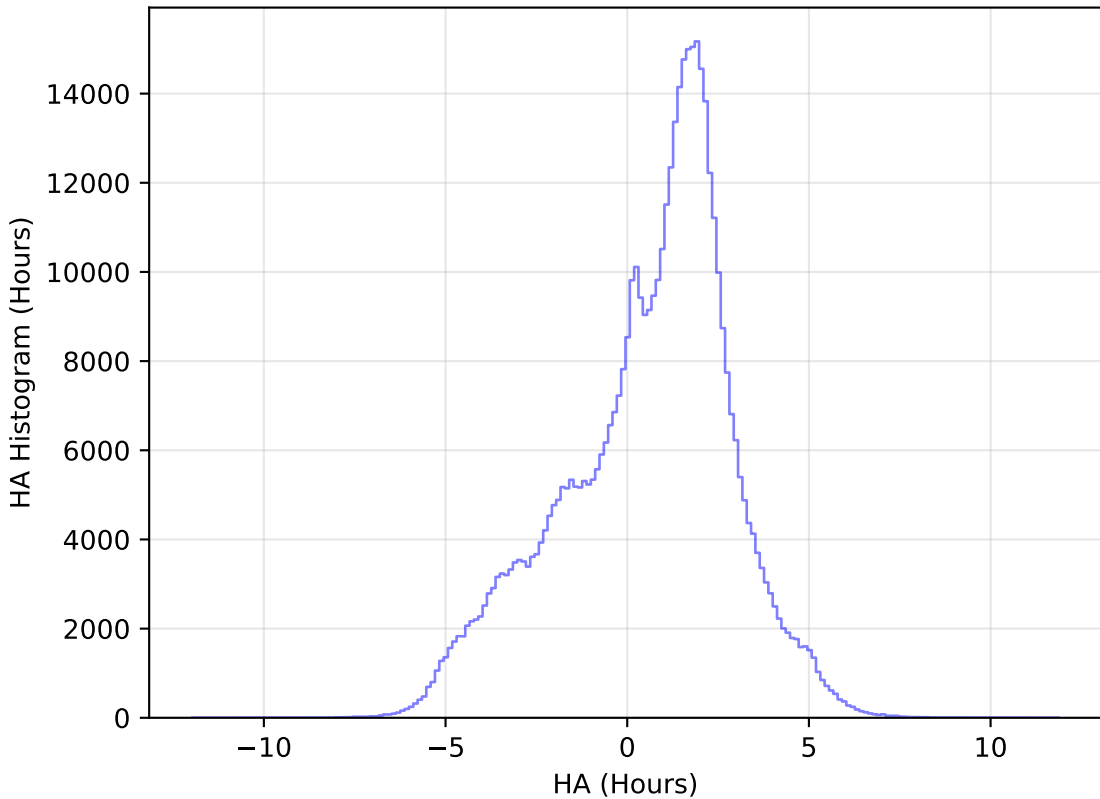
weather_cloudso36v3.4_10yrs All sky i band: HA Histogram
