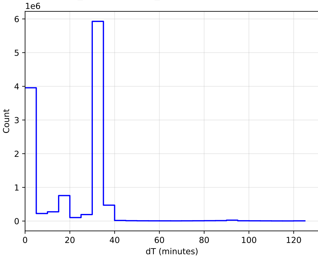
weather_cloudso36v3.4_10yrs WFD: DeltaT Histogram
