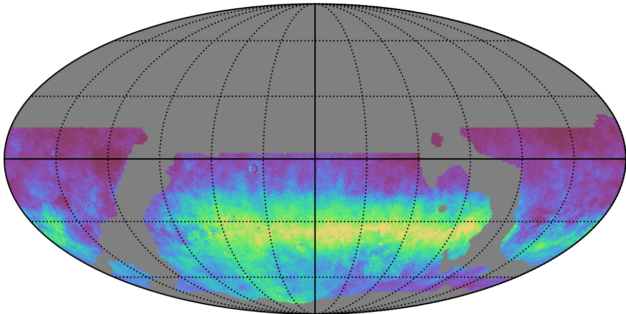
weather_cloudso36v3.4_10yrs WFD z band: AngleRms rotSkyPos
