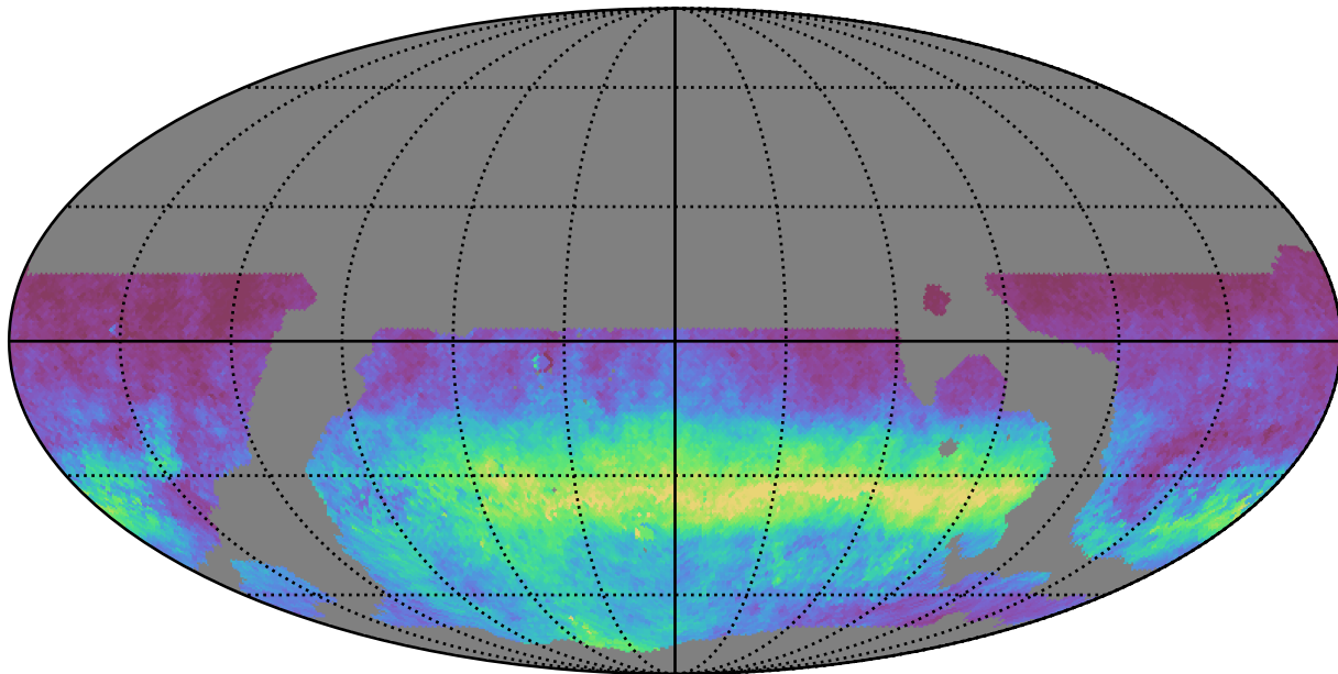
weather_cloudso36v3.4_10yrs WFD i band: AngleRms rotSkyPos
