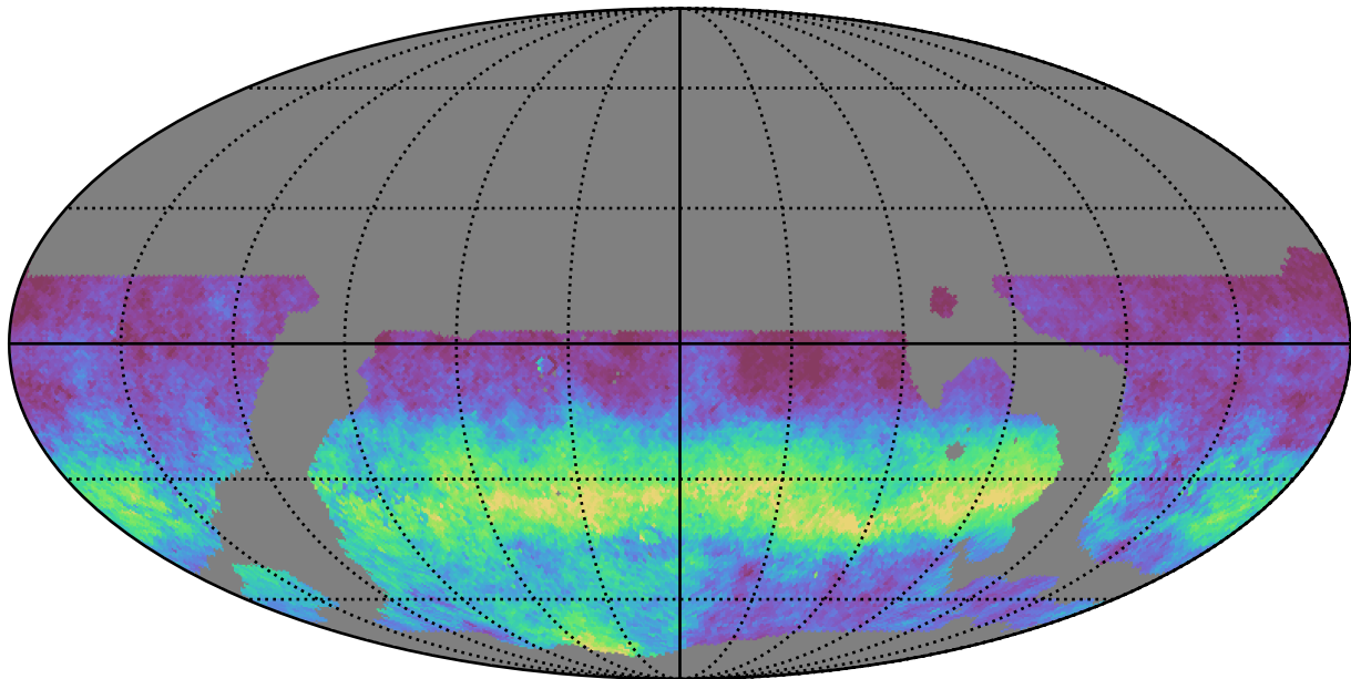
weather_cloudso36v3.4_10yrs WFD g band: AngleRms rotSkyPos
