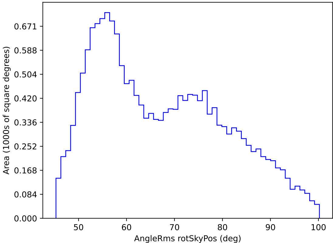
weather_cloudso36v3.4_10yrs WFD g band: AngleRms rotSkyPos
